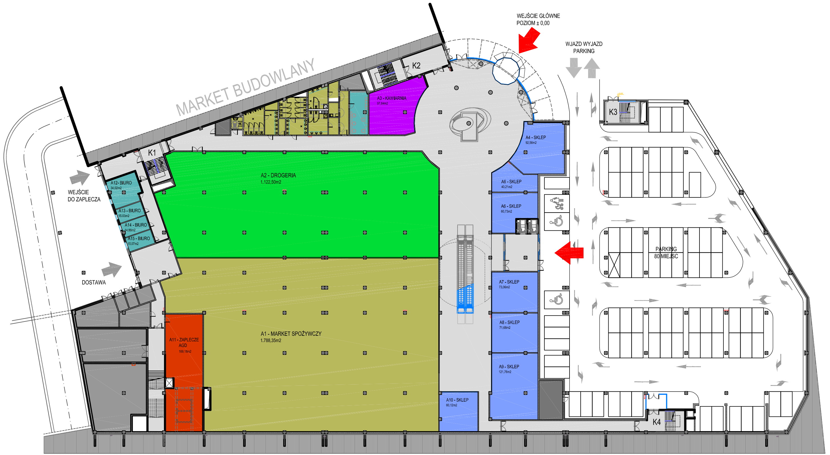
A - RZUT POZIOMU ± 0,00 - PARTER
